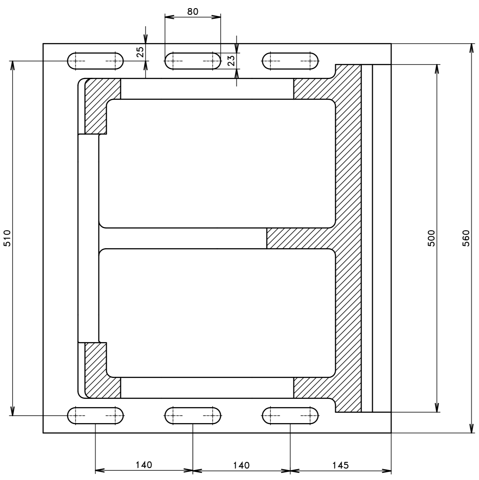
ŘEZ A-A
