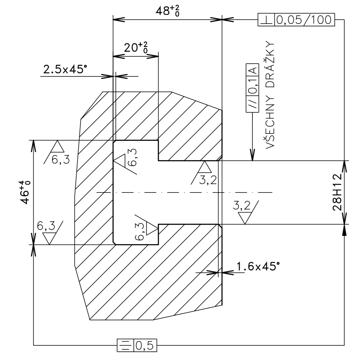
DETAIL D M 1:1
